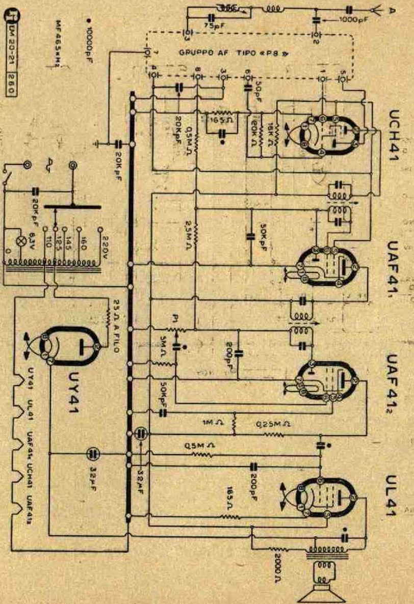
Lo schema elettrico del ricevitore.
